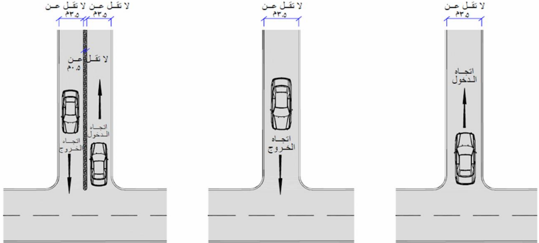
شكل (4) الحد الأدنى لإبعاد مداخل ومخارج مواقف السيارات السطحية
