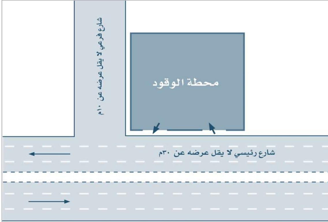
شكل رقم (3-4): تقاطع شارع مخصص للاستخدام التجاري لا يقل عرضه عن (٣٠ م) مع شارع فرعي
