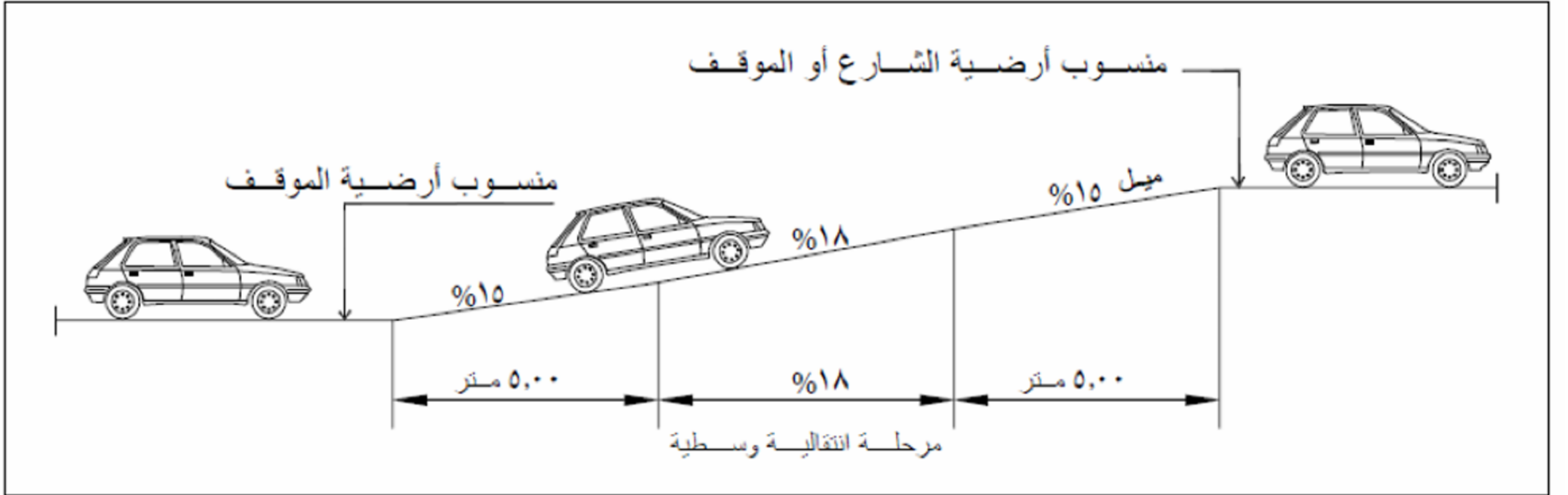
شكل (7) المنحدر المستقيم ومراحله الانتقالية.
